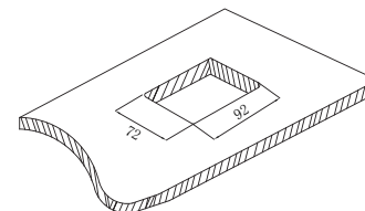
桌面安装方式开孔尺寸图 (单位：mm)
